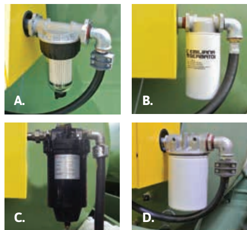
A. Filtro Clear Captor para agua µ30 o impurezas µ5. Filtro Clear Captor para água µ30 ou impurezas µ5. B. Filtro de absorción de agua 60 l/min µ30. Filtro de absorção de água 60 L/min µ30. C. Filtro de absorción de agua e impurezas de elevada capacidad µ25. Filtro de absorção de água e impurezas de alta capacidade µ25. D. Filtro para impurezas µ10. Filtro para impurezas µ10.
